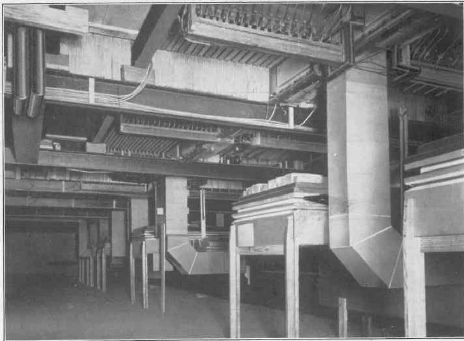
Magazingebläse im Innern der Orgel
