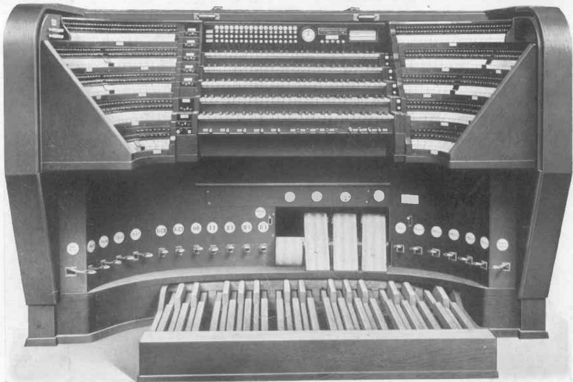
Rein elektr. fahrbarer Spielfisch 5 Manuale, 130 Register
